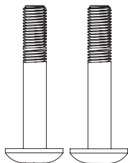
Болт (М8*55*13) 2 шт.
